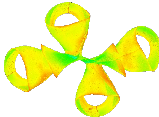
Flan1565 - 1564794 nodes
